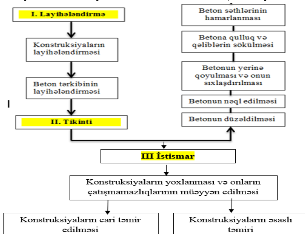
Şəkil 1. Monolit dəmirbeton işlərinin yerinə yetirilməsi fazası və mərhələləri
